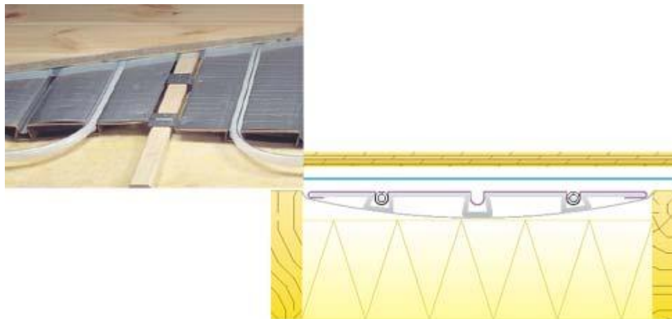
Figur 11. Gulvvarmeslanger nedlagt i selvbærende varmefordelingsplader. Kilde: Unopor Wirsbo A/S
