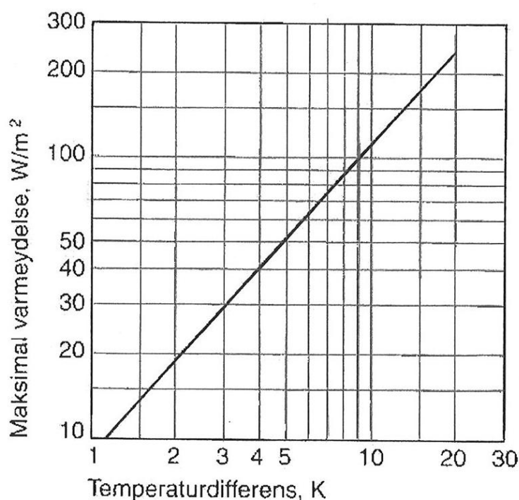
Figur 2. Kurven viser varmeydelse i forhold til temperaturdifferens.
