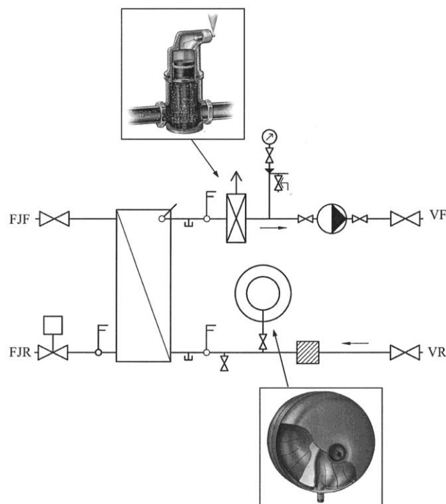
Figur 19. Microbobleaflifter i en gulvvarmeinstallation sikrer god afluftning af anlægget.
