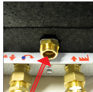
Cirkulationsstuds
